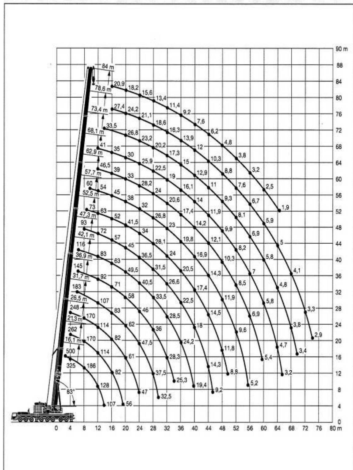
▲500 吨吊车 84 米主臂工况起升高度图
