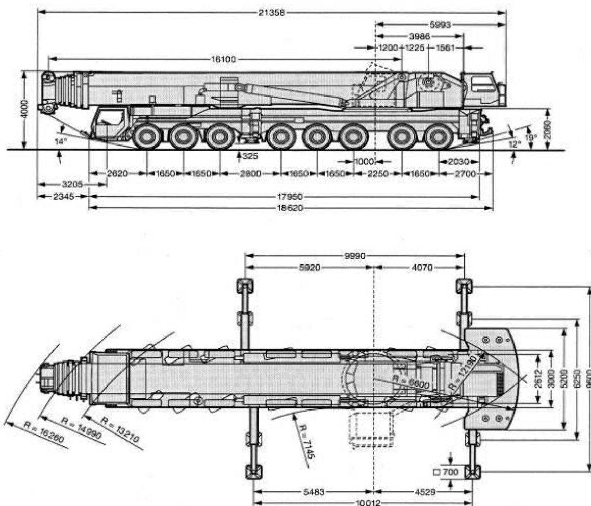
▲外形尺寸图
